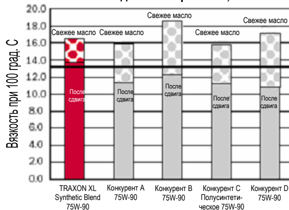
Сравнительный анализ вязкостей свежего масла и после испытания на сдвиг KRL при 100°C, GL-5 75W-90
